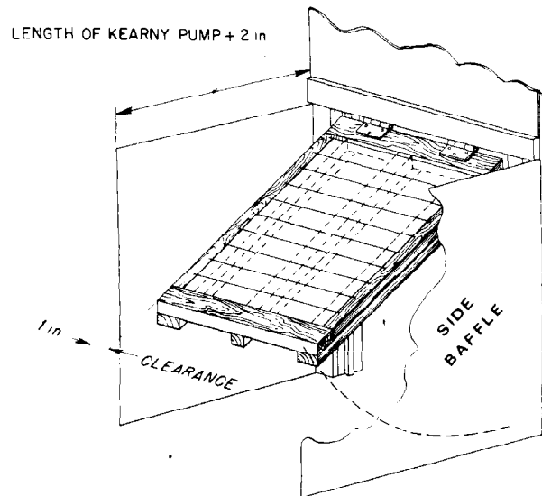
Fig. 25. Side baffles.
